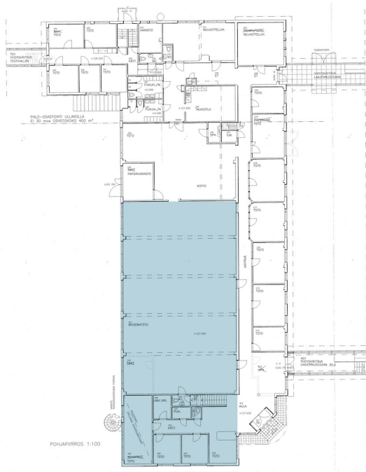
2.KERROS/ulokkaitat
